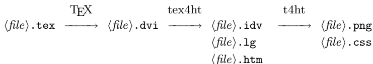
図 2.2 T E X4ht の動作の概要
