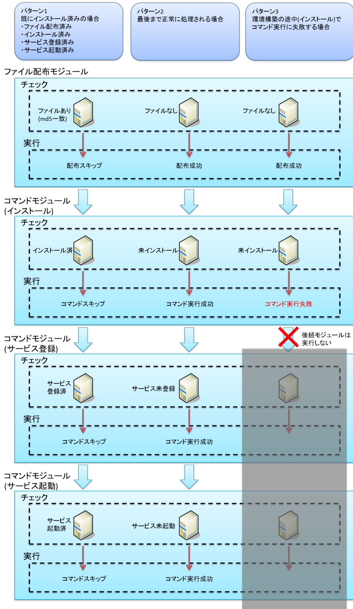
図 10-30 環境構築実行時のイメージ
