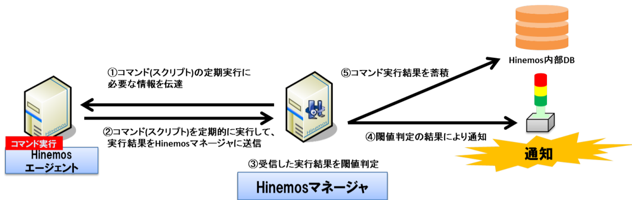
図 7-24 カスタム監視概要
