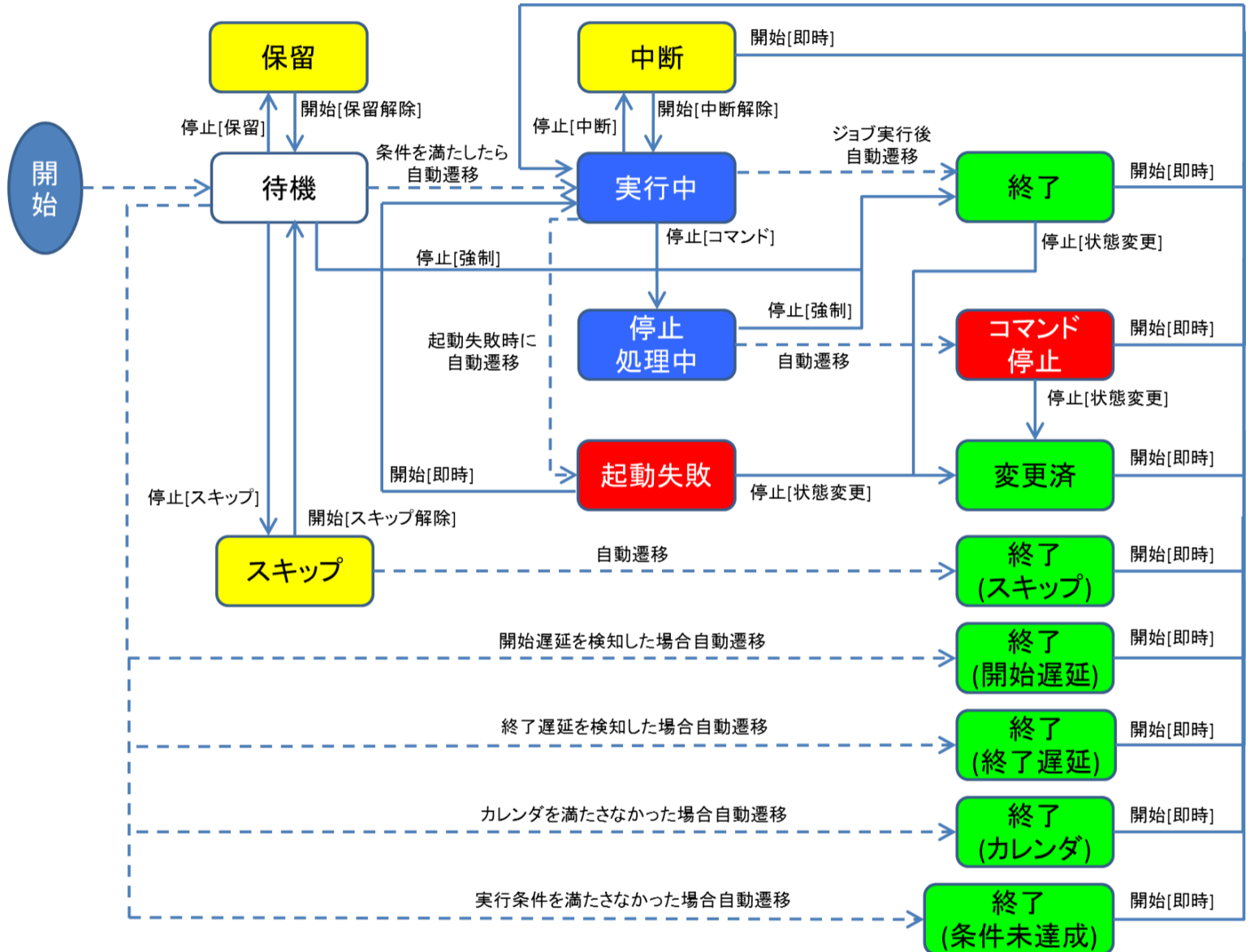
図 9-37 ステータス遷移図
