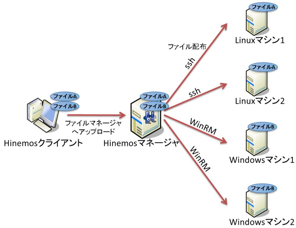
図 10-1 ファイル配布のイメージ
