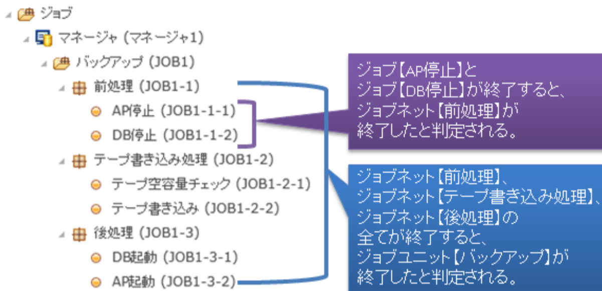
図 9-1 コマンドジョブ、ジョブネット、ジョブユニットの終了判定
