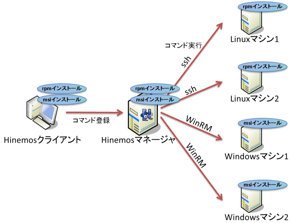
図 10-2 コマンド実行のイメージ
