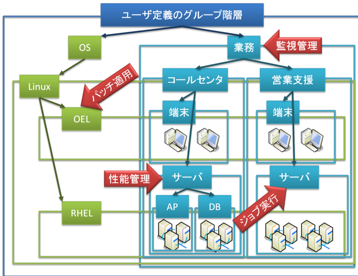
図 3-1 リポジトリのイメージ
