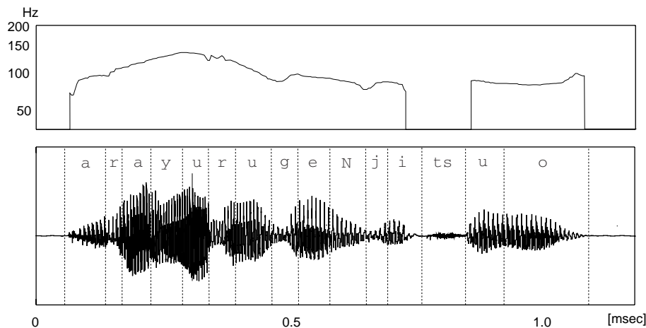
図5 ピッチ抽出とセグメンテーションの結果 (文章: あらゆる現実を...)
