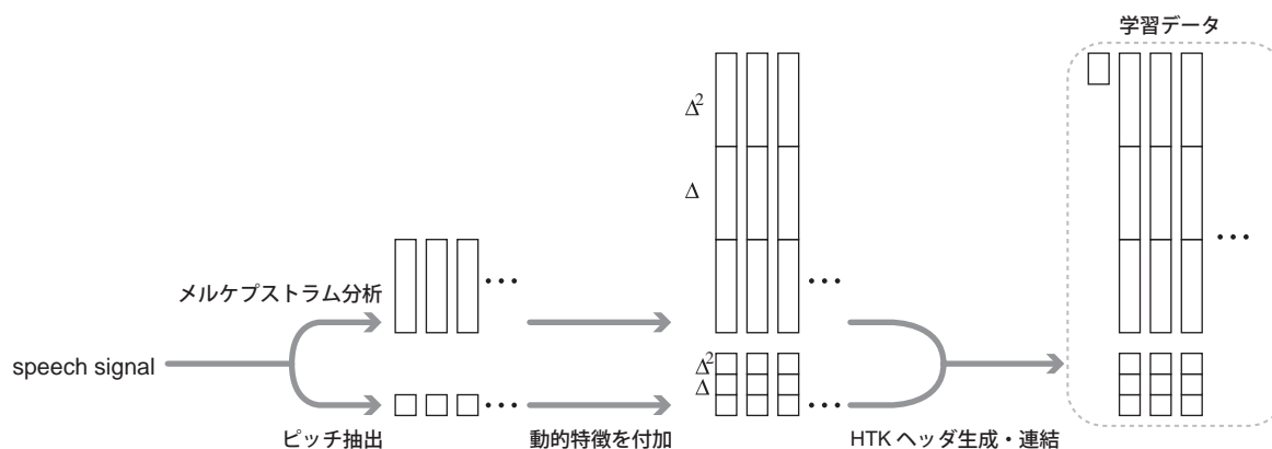
図6 特徴ベクトルの構成
