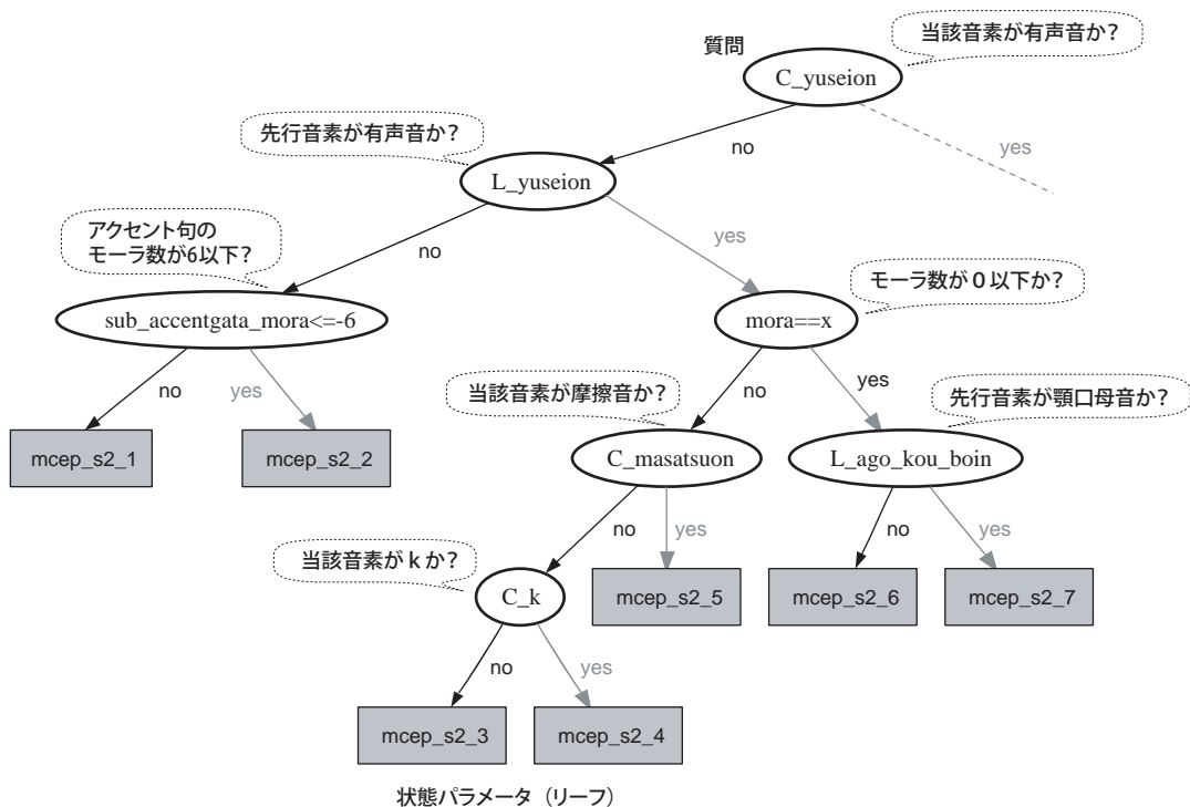
図8 モデル学習によって作成された木構造の一部
