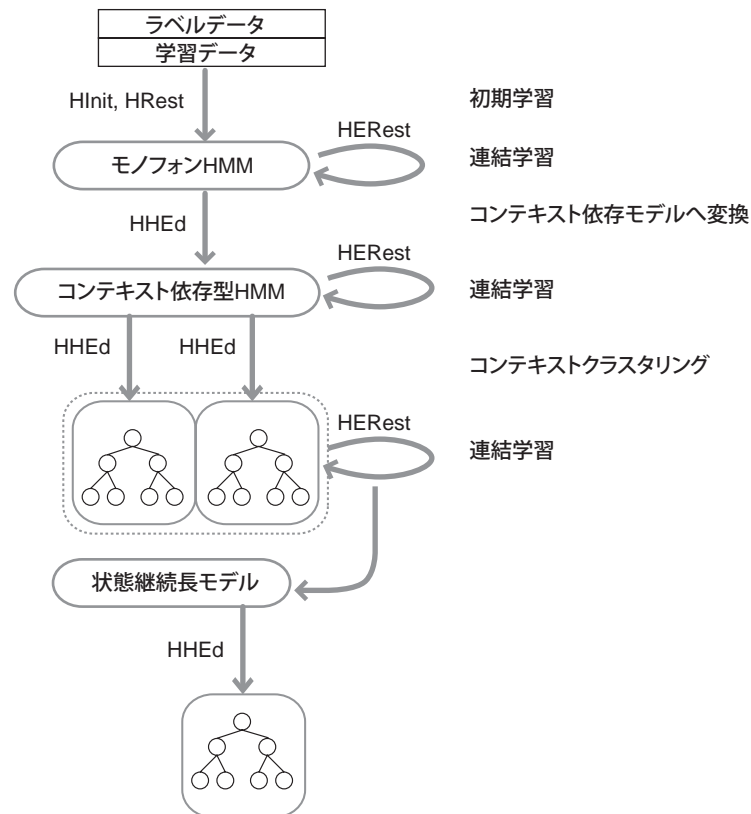
図7 モデル学習の過程
