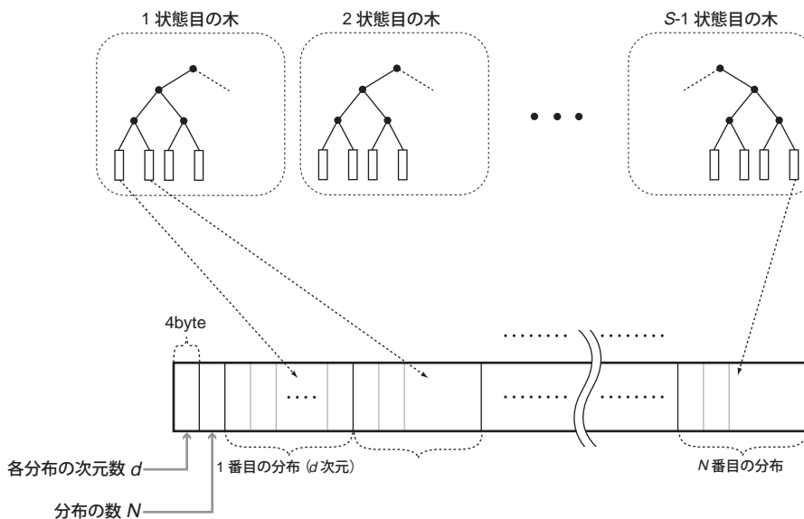
図9 Galatea Talk 用音響モデルの構造
