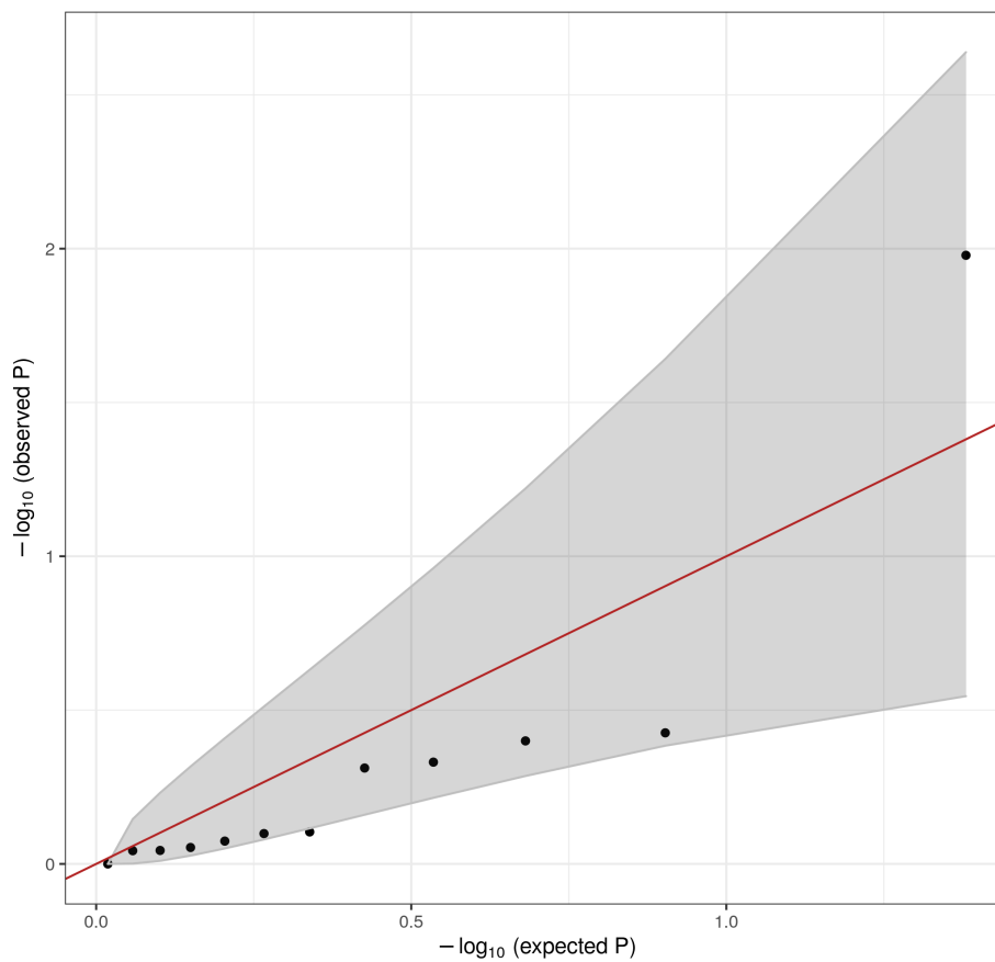
\theta Q-Q plot: TIMMDC1 (site 119)
