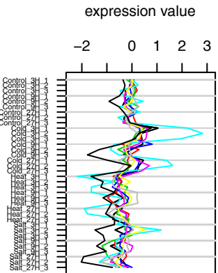
Cluster 1 ( 9 genes )
