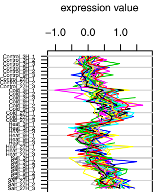
Cluster 7 ( 35 genes )
