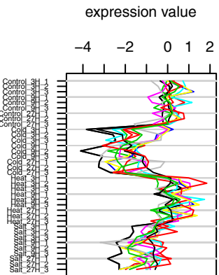
Cluster 2 ( 11 genes )
