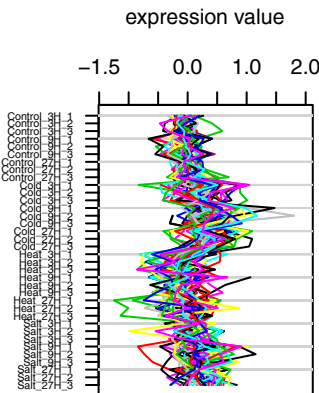
Cluster 5 ( 54 genes )
