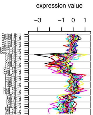
Cluster 9 ( 42 genes )
