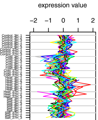
Cluster 8 ( 61 genes )
