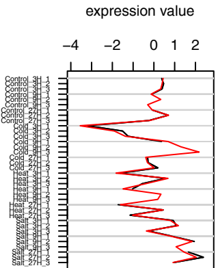
Cluster 4 ( 2 genes )
