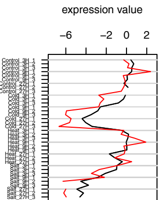
Cluster 3 ( 2 genes )
