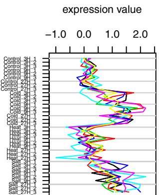
Cluster 6 ( 7 genes )
